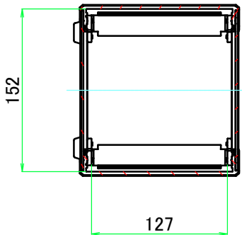
A-A ( 1 : 5 )
